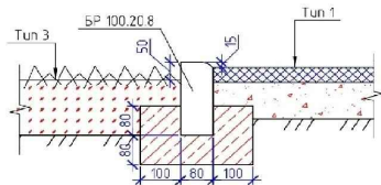
Сопряжение покрытий 1 - 3.
