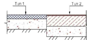
Сопряжение покрытий 2 - 3.
