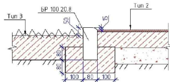
Сопряжение покрытий 2 - 3.
