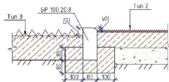
Сопряжение покрытий 2 - 3.
