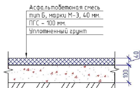
Асфальтобетонное покрытие (Тип 1)
