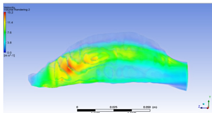
Рис. 2.5. Поле значений скорости течения воздуха в момент времени t = 1 (сценарий 25 °С) в носовой полости
